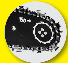
Крепление ведомой звездочки на 4-х заклепках: повышенная долговечность
