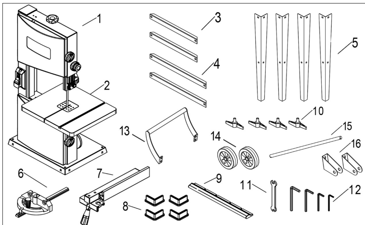
Рисунок 1. Комплектация для модели BELMASH WBS-254/2
