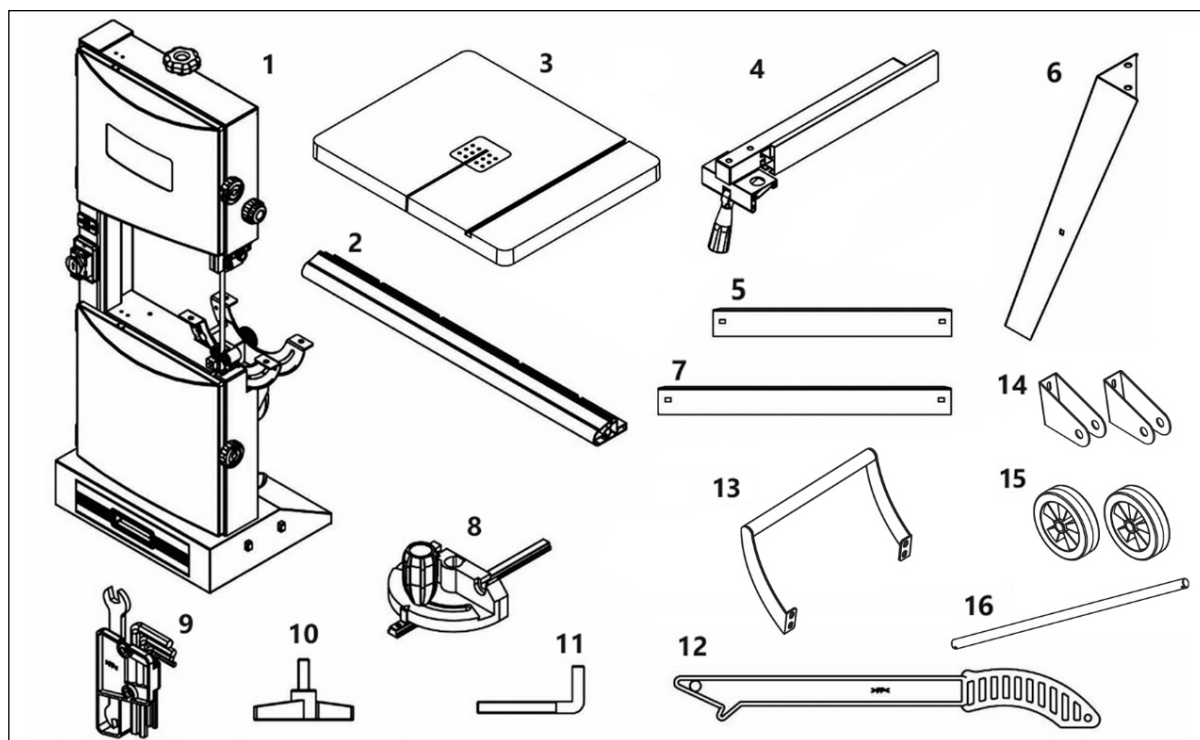
Рисунок 2. Комплектация для модели BELMASH WBS-254
